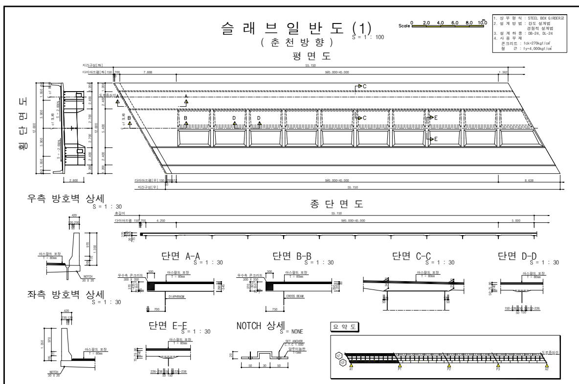
<그림 1.4> 조양교(양양) 슬래브 일반도
