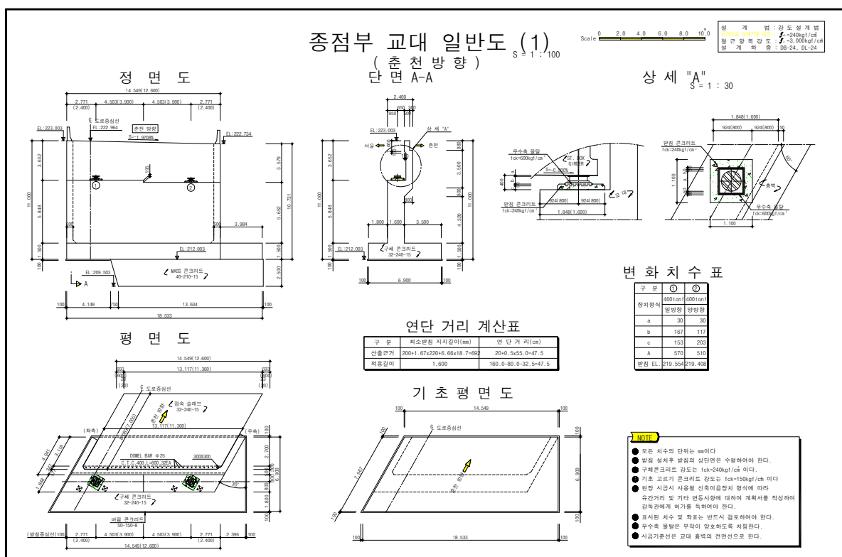
<그림 1.6> 조양교(양양) 종점교대 일반도
