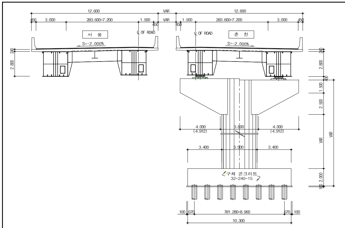
<그림 1.3> 조양교(양양) 횡단면도
