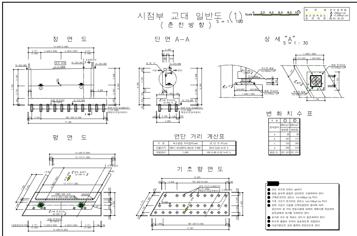
<그림 1.5> 조양교(양양) 시점교대 일반도
